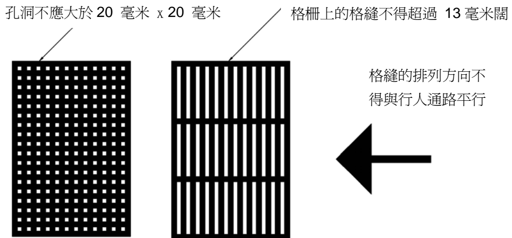
▲圖 1 - 格柵尺寸及方向
