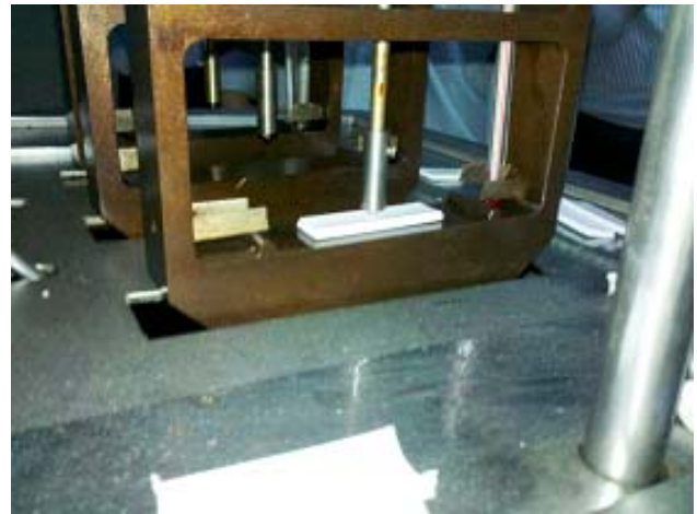
▲高溫針刺式測試塑膠之堅韌度
